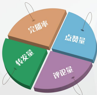
图7-10 数据加权
