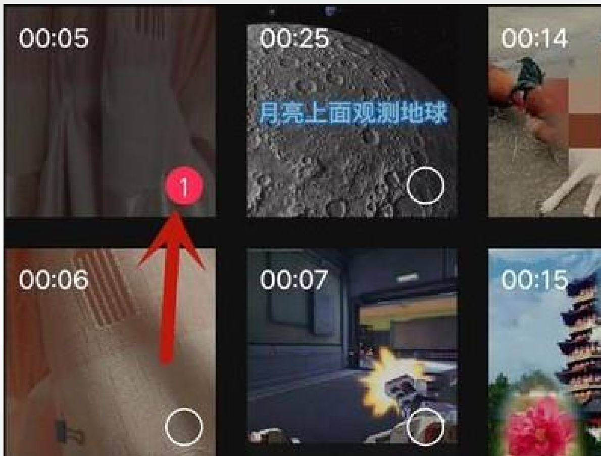
图4-7 选择视频
