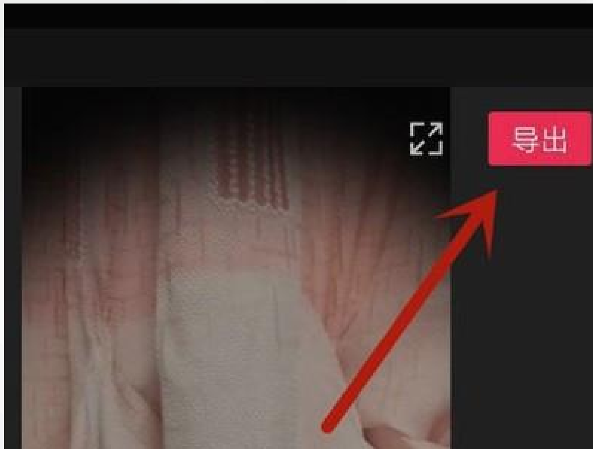
图4-11 导出视频
