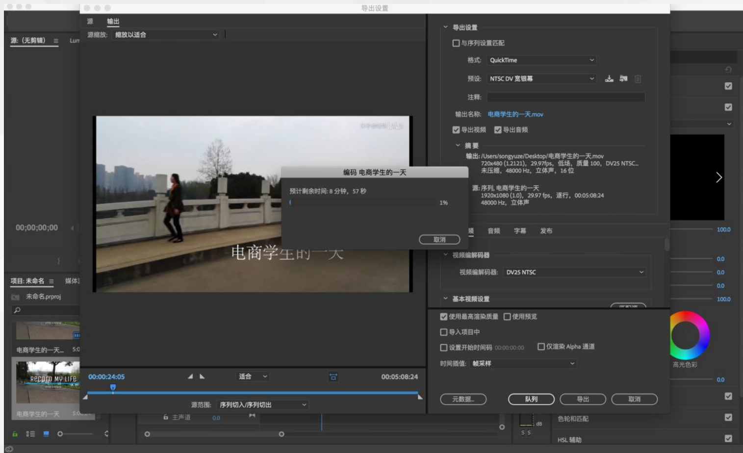
图4-5 导出视频
