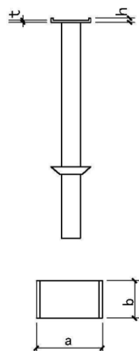
图 3 可调托撑构造图
