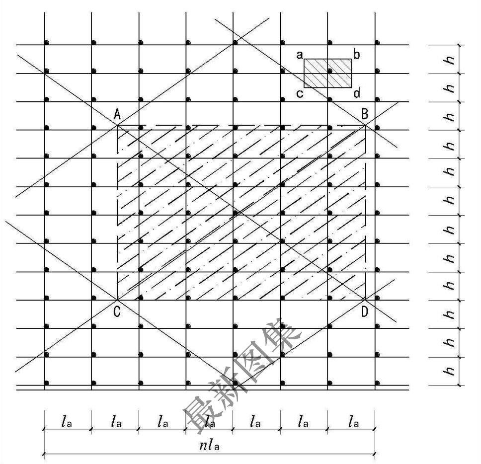
图 4 立杆承受的每米结构自重标准值计算图 为简化计算，双排脚手架立杆承受的每米结构自重标准值是采用内、外立杆的平均值。
