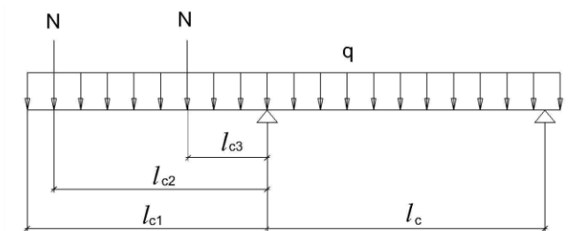
图 5.6.5 悬挑脚手架型钢悬挑梁计算示意图
