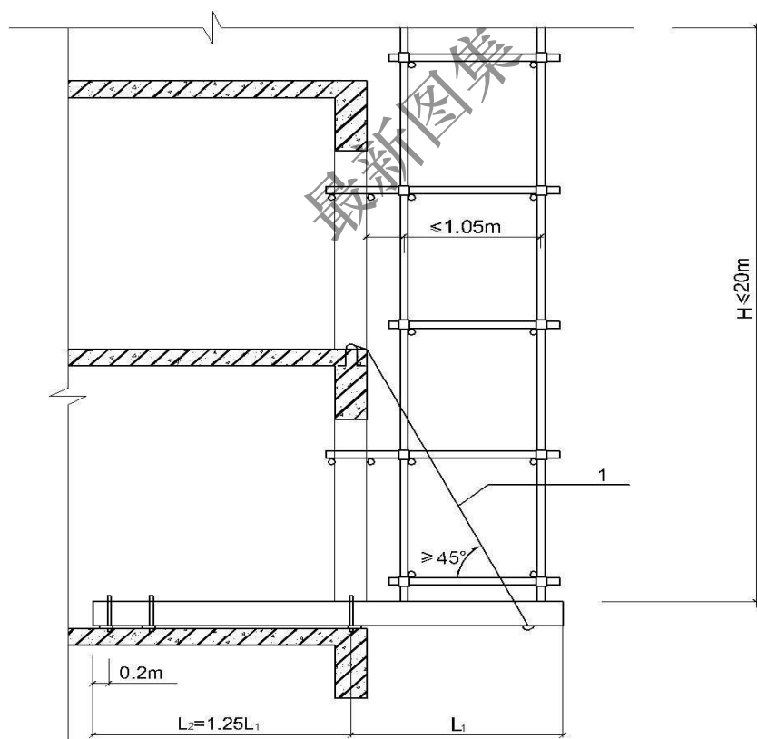
图 6.10.2 型钢悬挑脚手架构造
