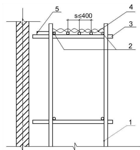
图 6.2.1-2 铺竹笆脚手板时纵向水平杆的构造
