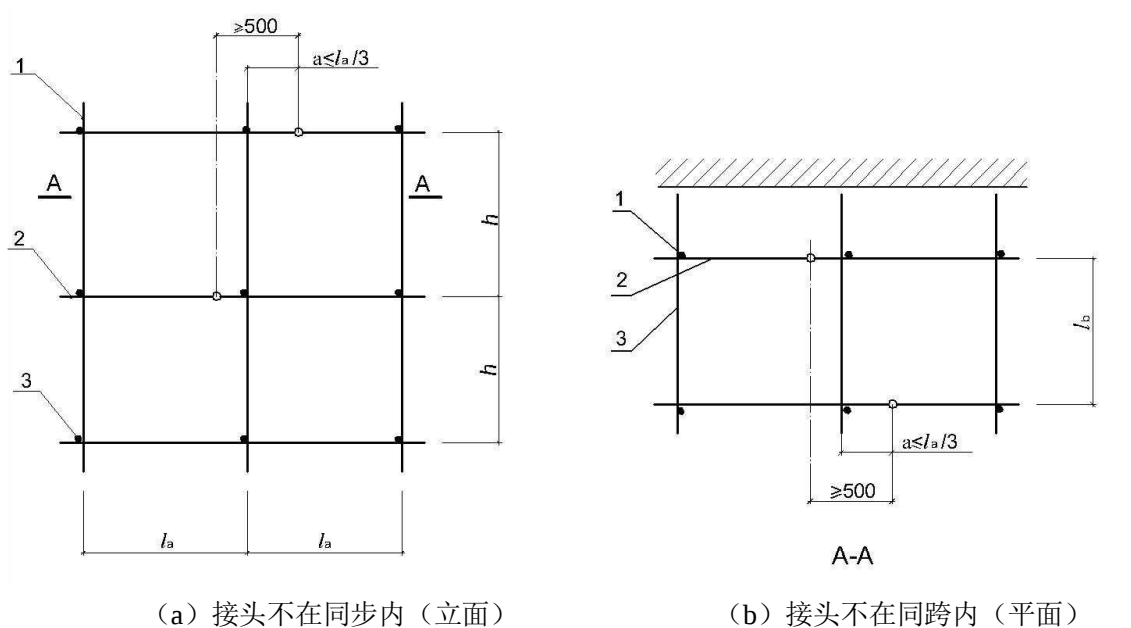
图 6.2.1-1 纵向水平杆对接接头布置
