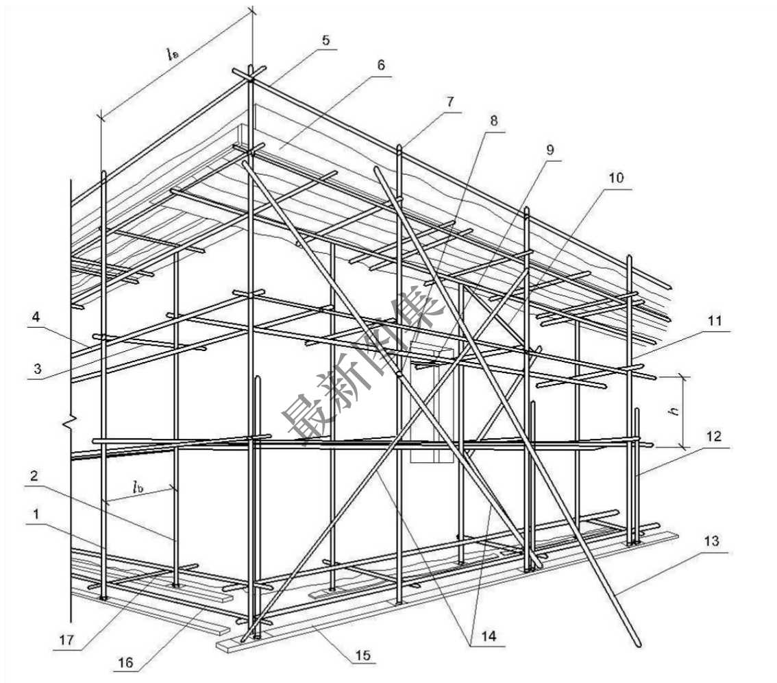
图 1 双排扣件式钢管脚手架各杆件位置
