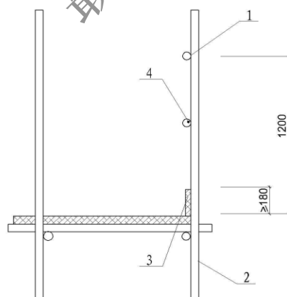
图 7.3.12 栏杆与挡脚板构造
