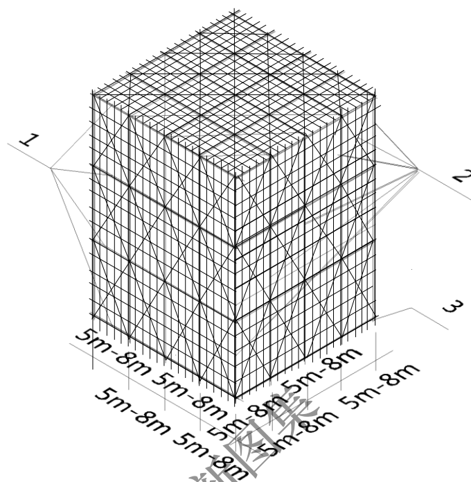
图 6.9.3-1 普通型水平、竖向剪刀撑布置图
