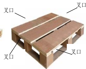
图 5-25 四向叉入型
