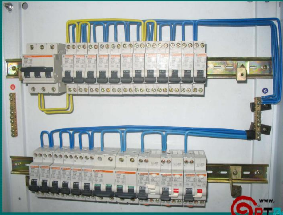
空开A相配线照片：
