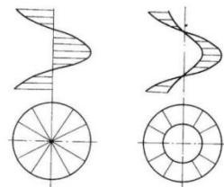
a)实心平螺旋面 b)空心平螺旋
