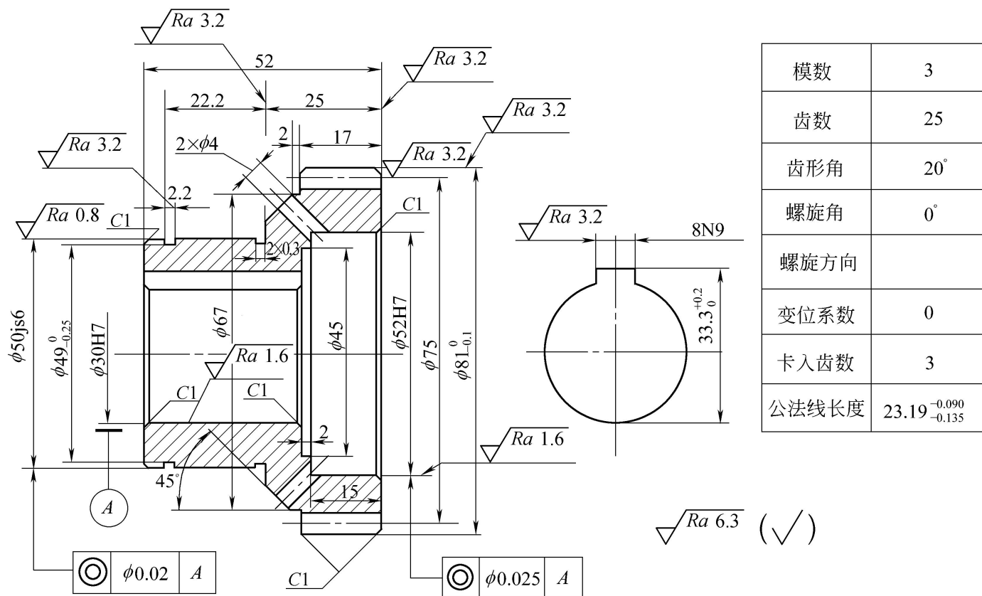
图9.2.2 套筒齿轮
