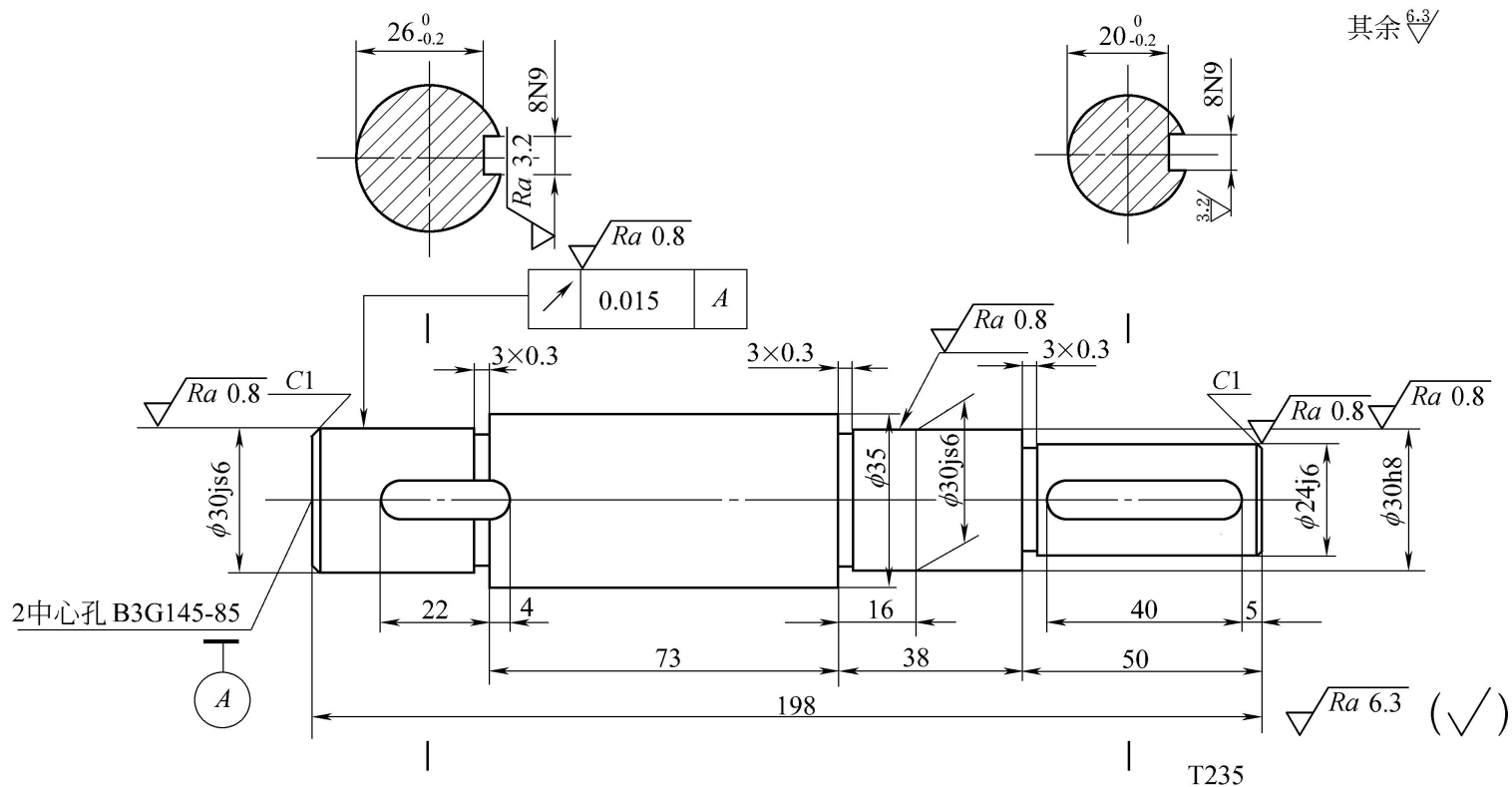
图9.2.1 轴
