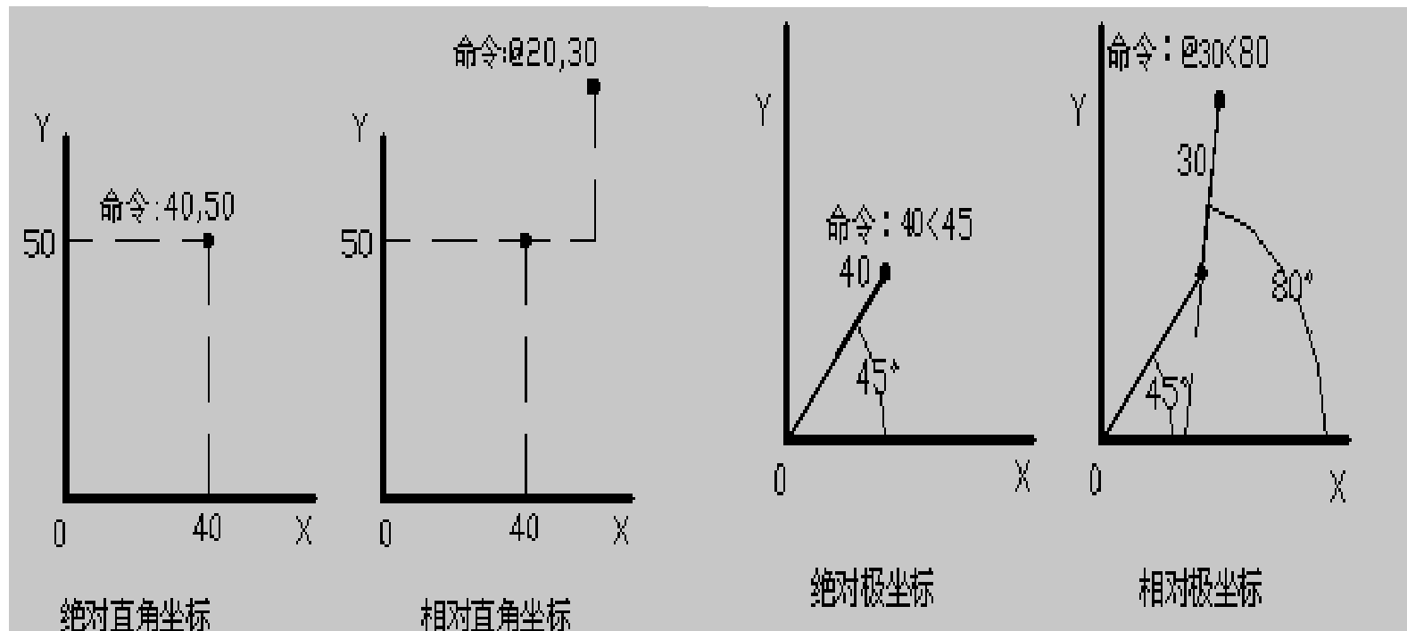
图2-3 AutoCAD坐标系
