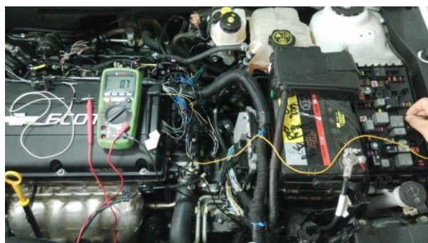
图 6-10 线路断路检查
