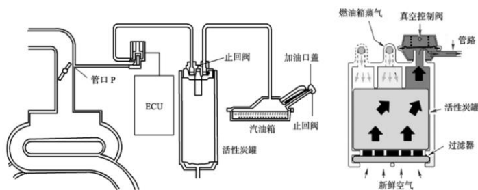
图 6-3 活性炭罐
