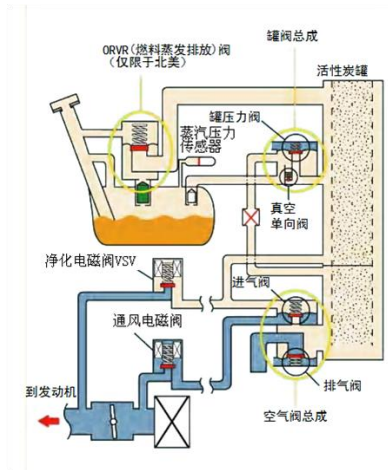
图 6-6 丰田汽车上的 EVAP 系统
