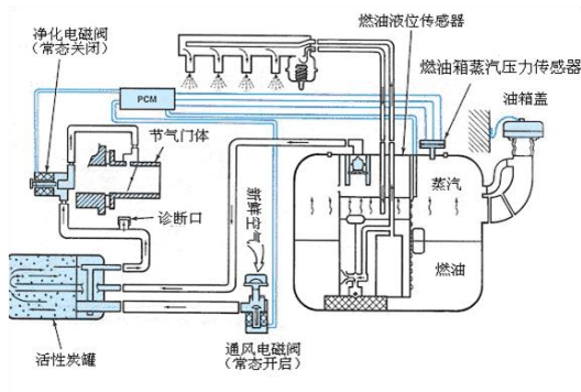
图 6-5 通用汽车上的加强型 EVAP 系统
