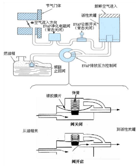
图 6-4 非加强型 EVAP 系统
