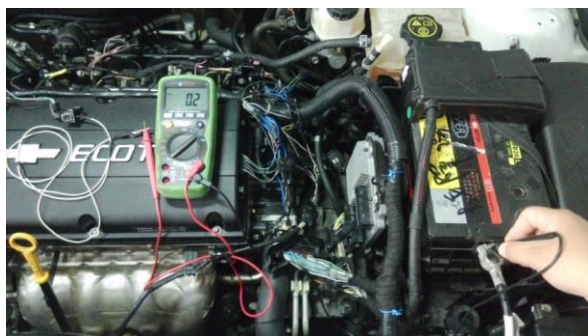
图 6-13 线路短路检查
