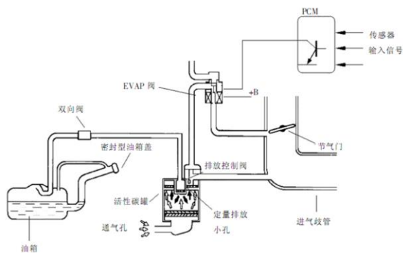
图 6-2 燃油蒸发控制系统示意图
