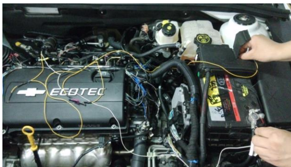
图 6-19 Q12 蒸发排放吹洗电磁阀检查
