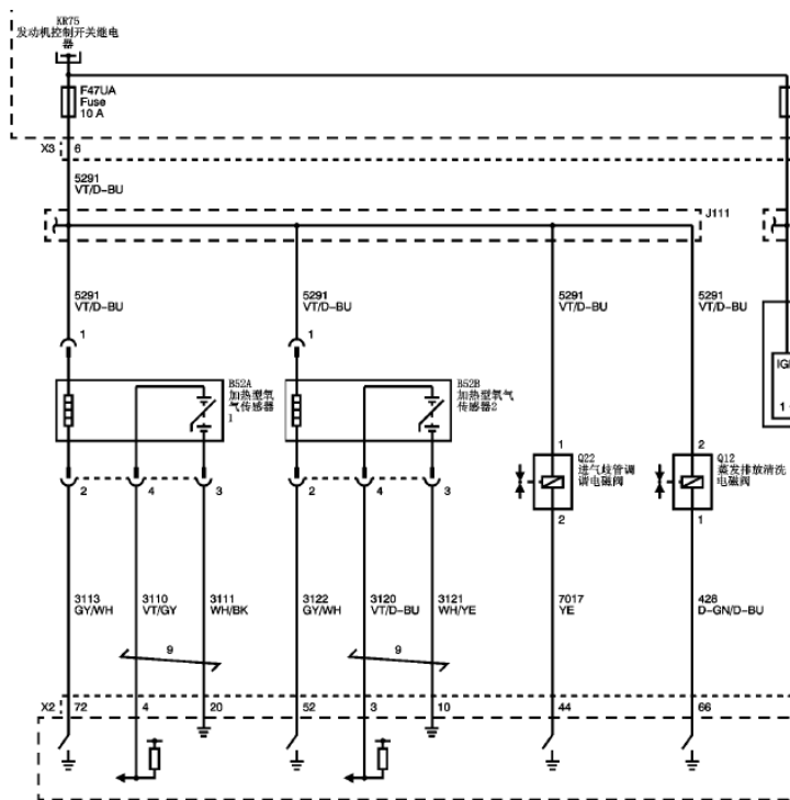
图 6-8 蒸发排放吹洗电磁阀系统电路图
