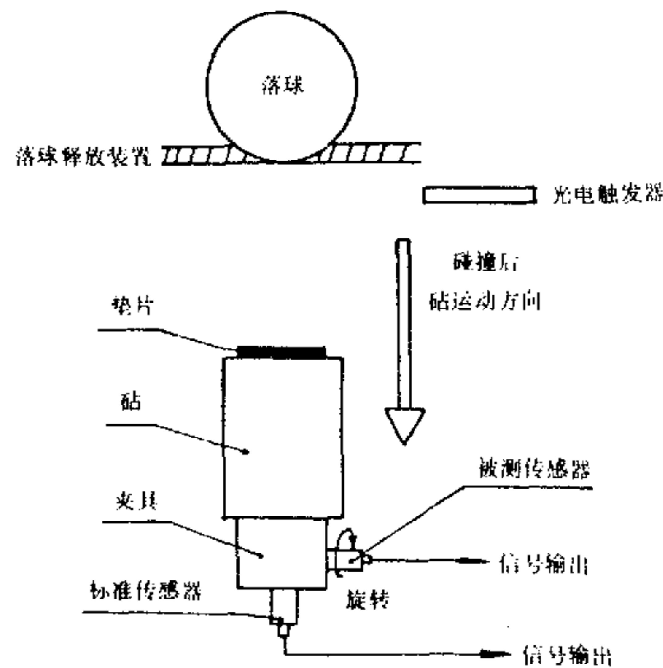
横向冲击灵敏度测试设备原理图
