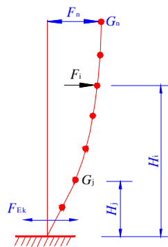
图 5.2.5 结构水平地震作用计算简图
